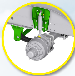
Suspension hydraulique du timon et des essieux
